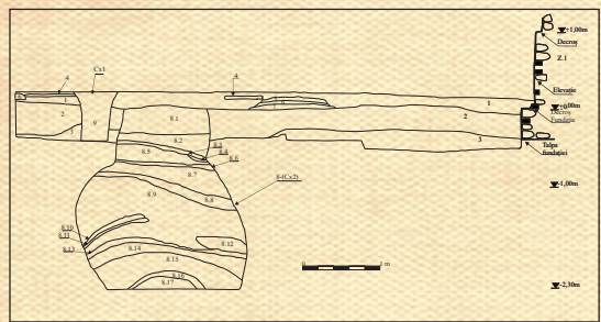
Groapa de provizii: imagine generală și secțiune Vorratsgrube: Gesamtansicht und Grundriss
